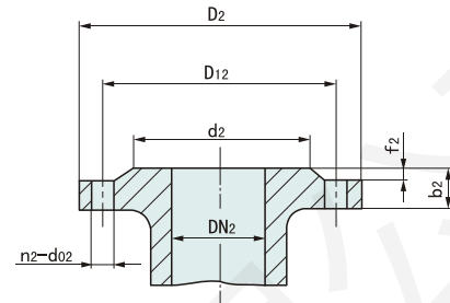
吐出口法兰 Outlet flange
