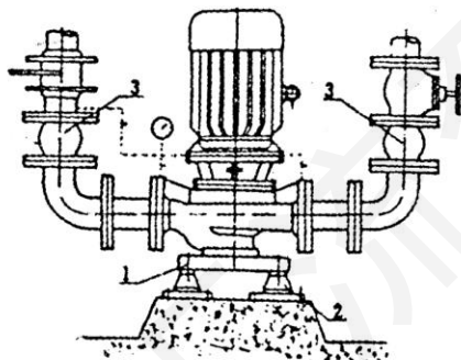
2. 配 KL 联接板, 加隔振器安装
