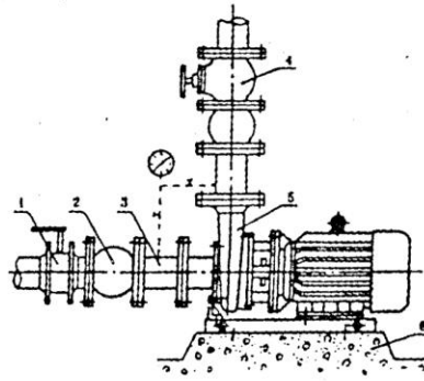
加隔振器安装
