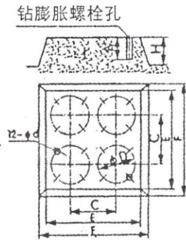
柔性联接基础图
