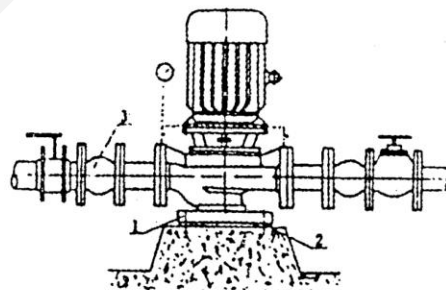
1. 配 KL 型联接板, 加隔振器安装
