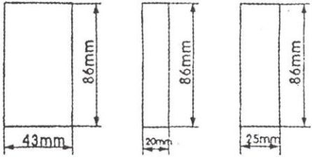
SD 型隔振垫 0.5 基本块尺寸
