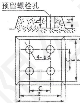
硬性联接基础图
