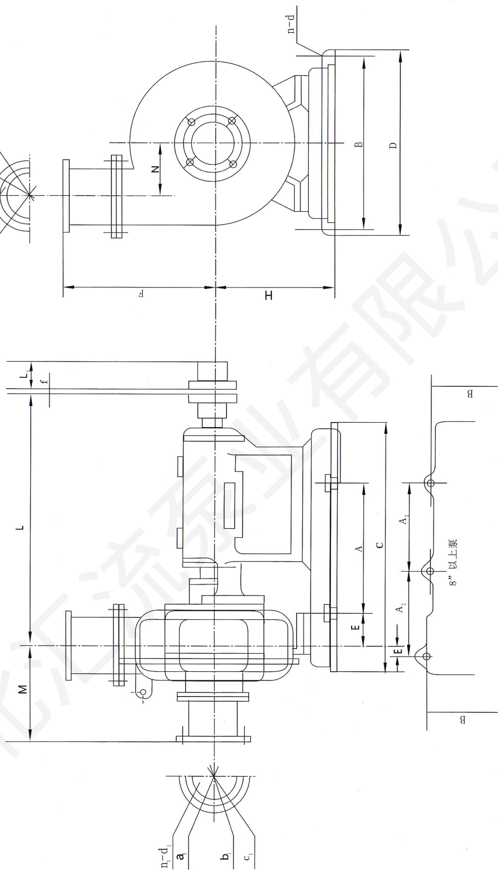
4、6、8、10、12PN 型泵外形图
