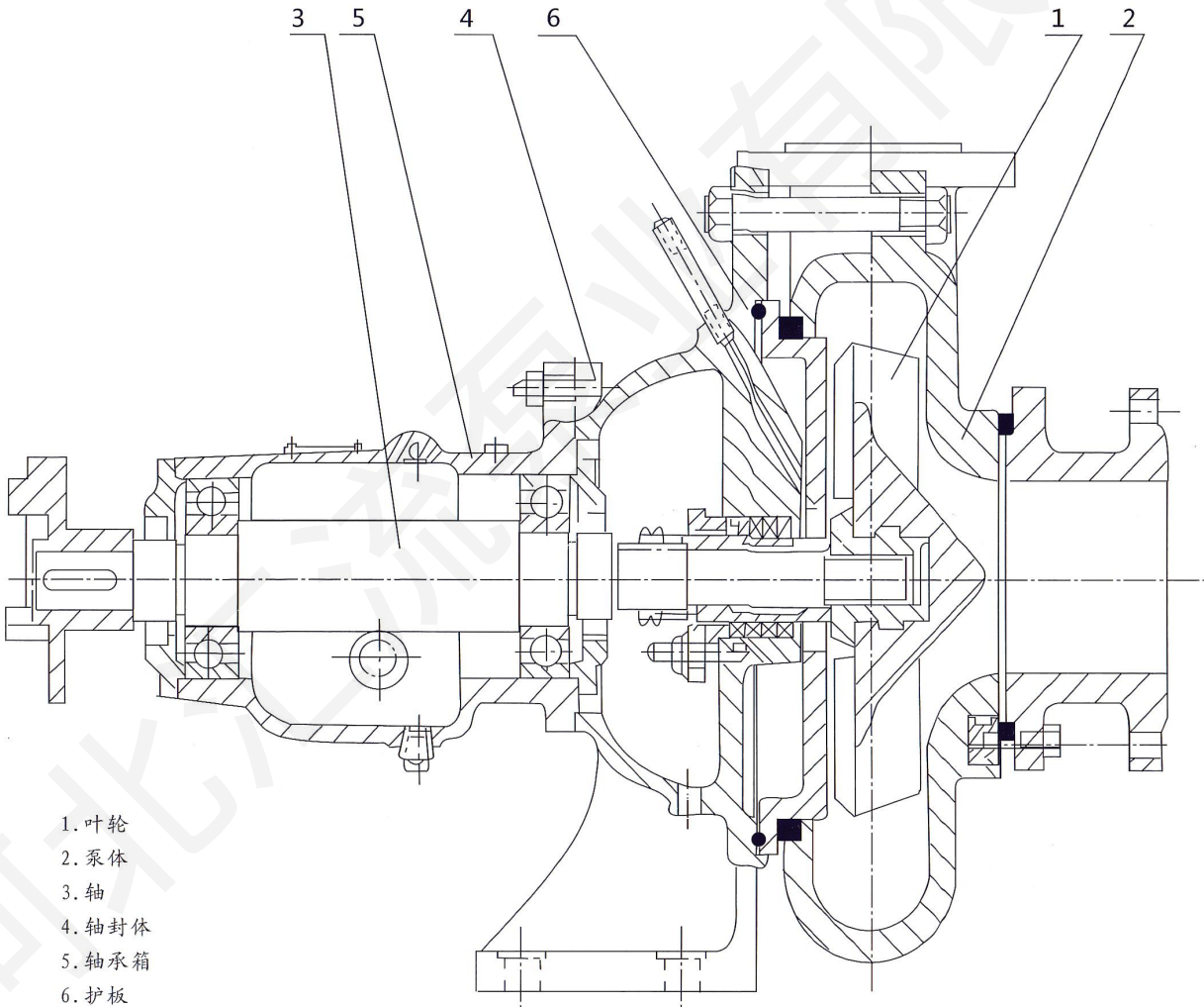
1、2、3 PN 型泵结构图
