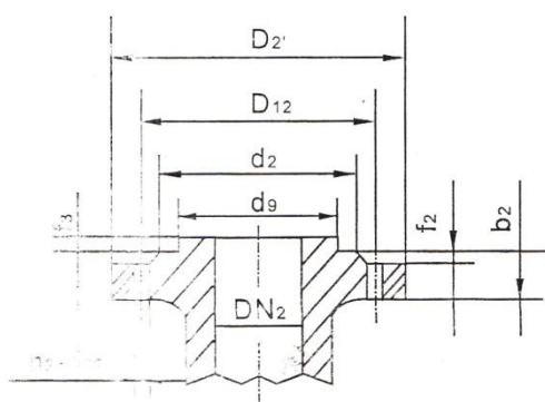
吐出口法兰
