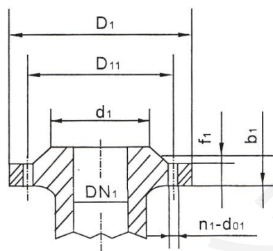
吸入口法兰
